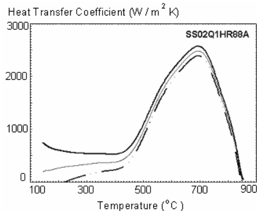
Fig. 11. Actual Heat Transfer Coefficient Graph.
