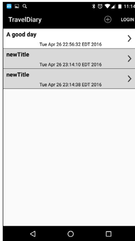
MainActivity
